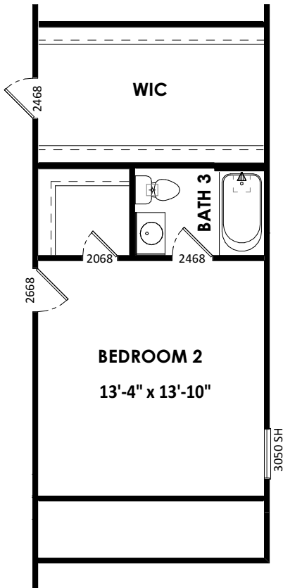
BEDROOM 2 SUITE
