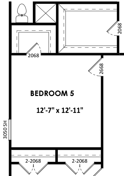
BEDROOM 5
